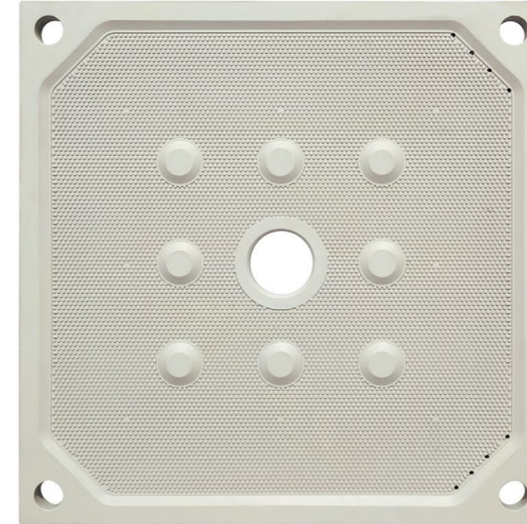
1500 型高温高压厢式滤板
