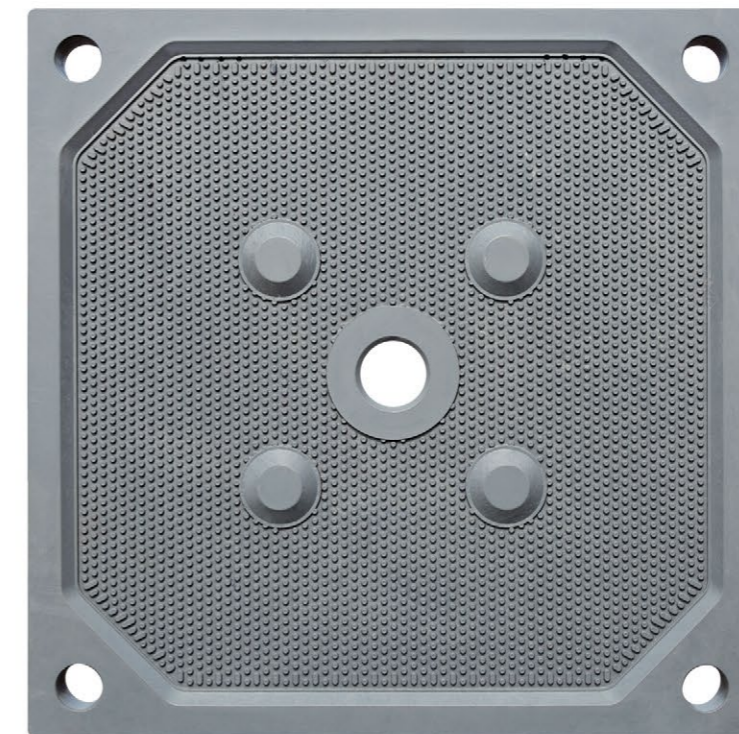
1000 型厢式滤板
