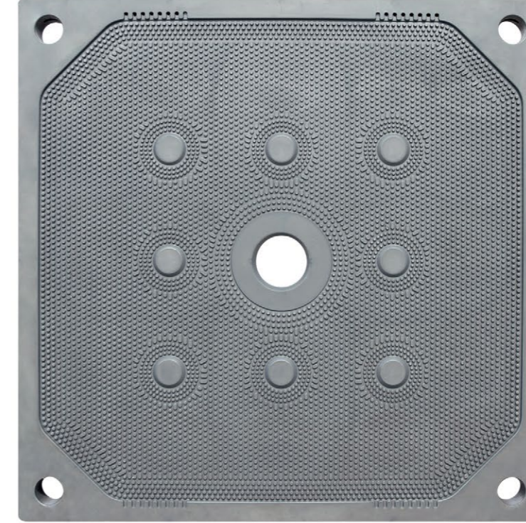
1250 型隔膜滤板
