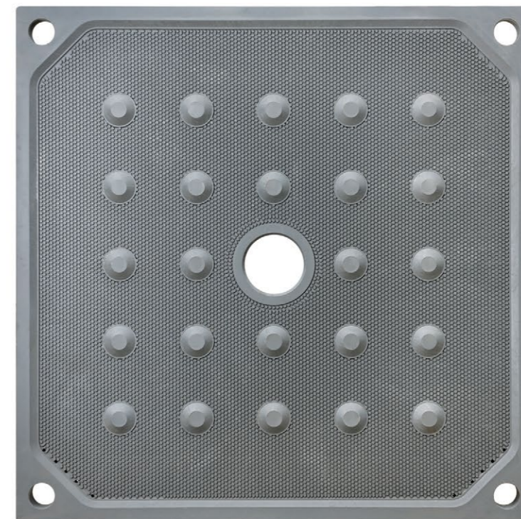
2000 型厢式滤板
