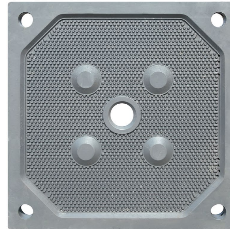
870 型厢式滤板
