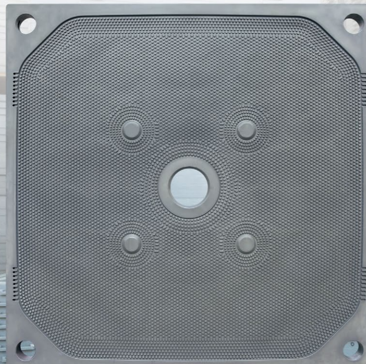
2000×2000 注塑膜片
