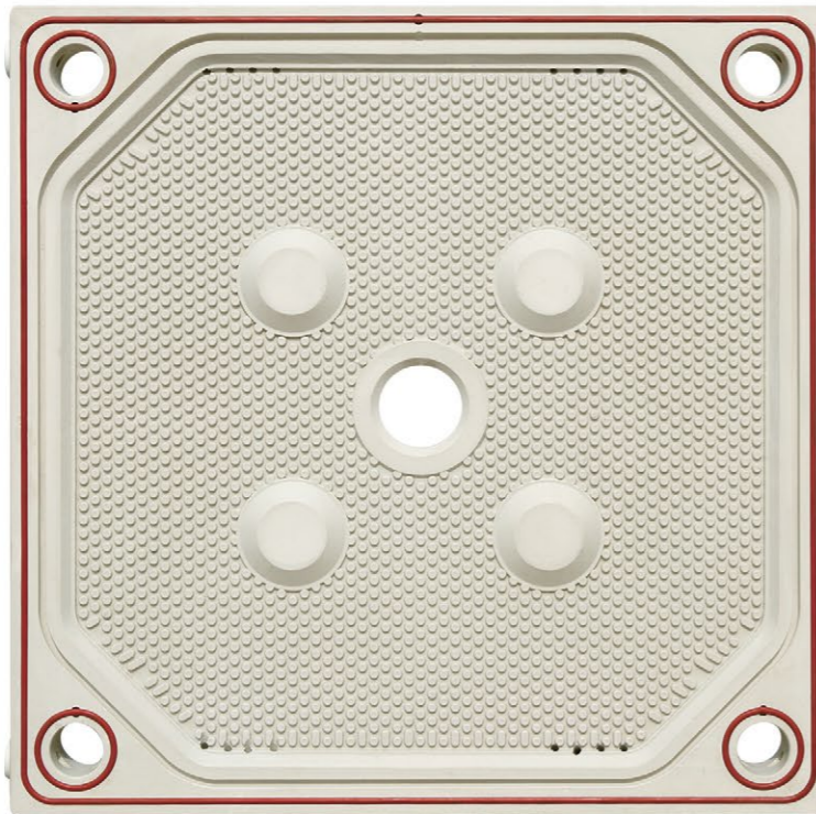
1000 型密闭高温高压厢式滤板
