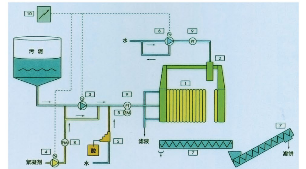
1、压滤机；2、滤布洗涤系统；3压滤机进料泵；4、高分子电解质计量泵；5、酸洗泵；6、高压滤布洗涤泵；7、滤饼输送机；8、流量计；9、压力传感器；10、PLC（可编程逻辑控制器）
