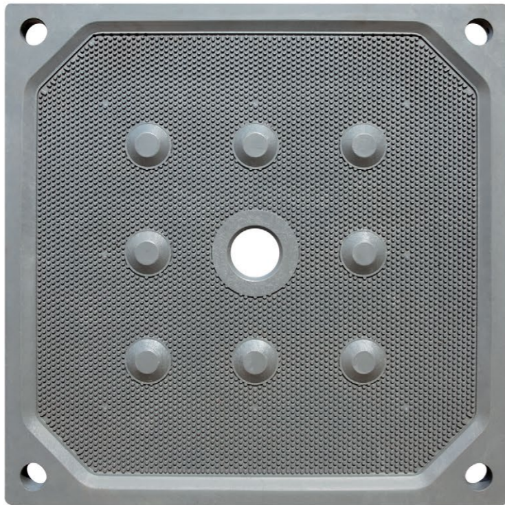
1500 型厢式滤板
