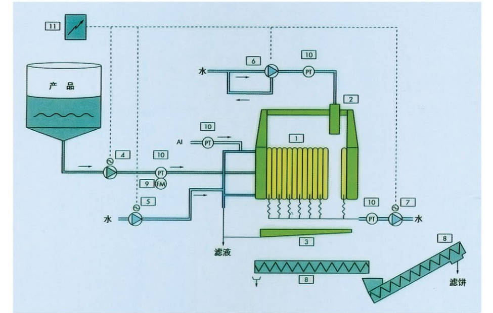
1、压滤机；2、滤布洗涤系统 3、落盘；4、压滤机进料泵；5、滤饼洗涤泵；6、高压滤布洗涤泵；7、隔膜板挤压泵；8、滤饼输送机；9、流量计；10、压力传感器；11、PLC（可编程逻辑控制器）
