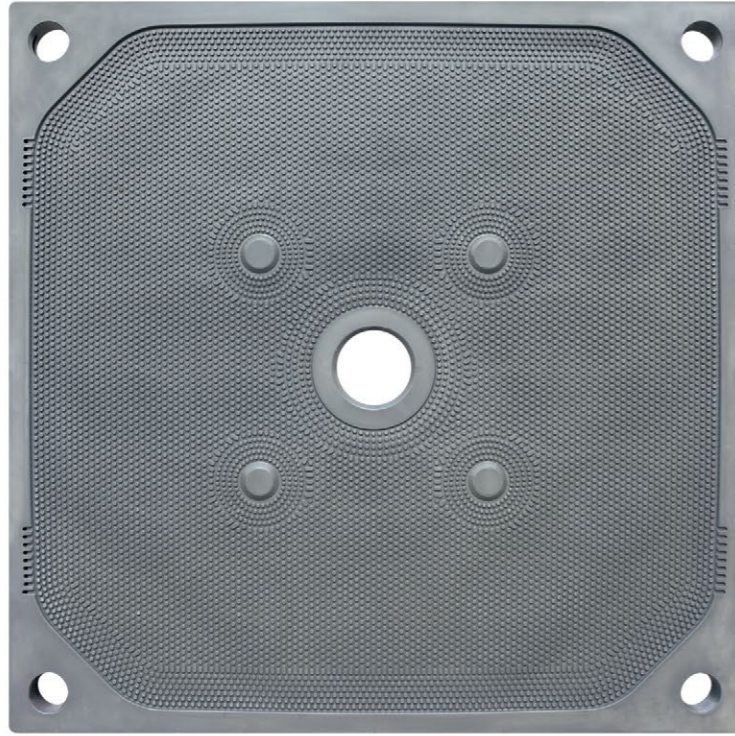
1500 型隔膜滤板
