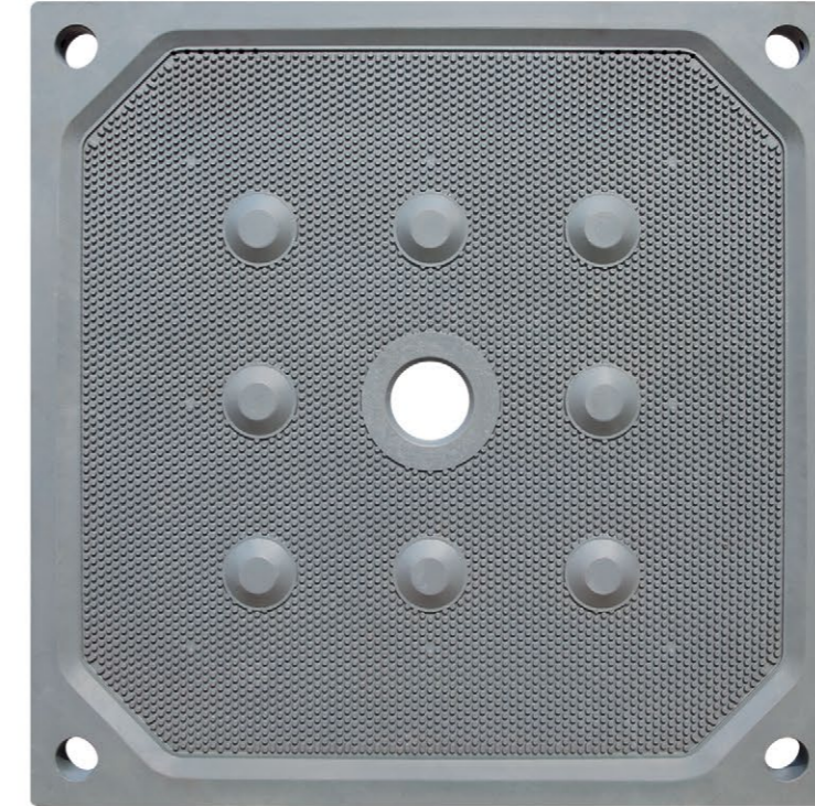
1250 型厢式滤板
